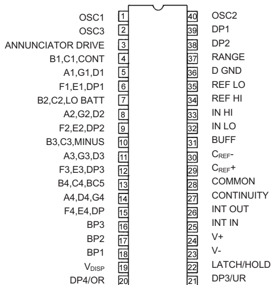
ICL7129CPL
