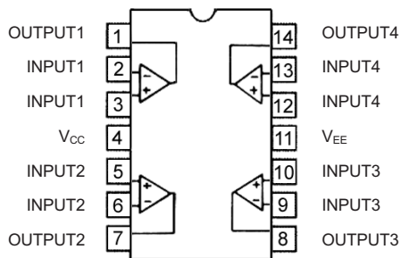
MC33174P
