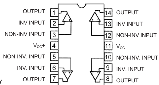
TL044
