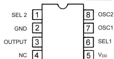
UM3561A
