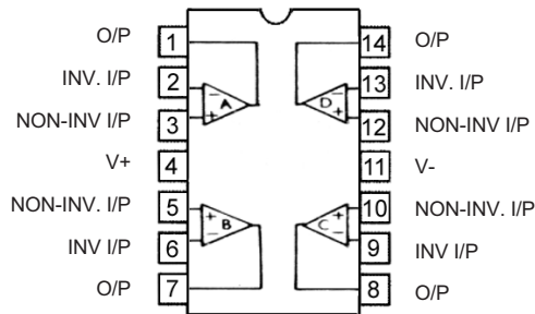
LM324N
