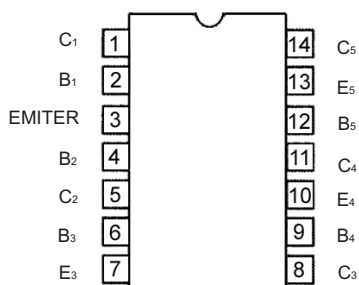
CA3086
