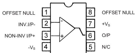
OP07CN
