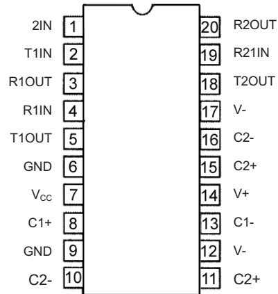
MAX233
