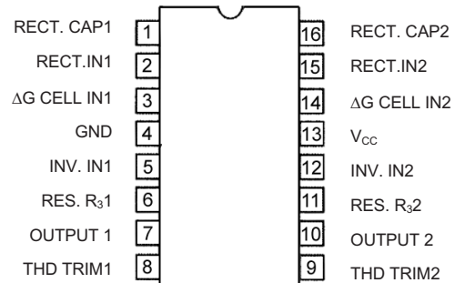
NE571
