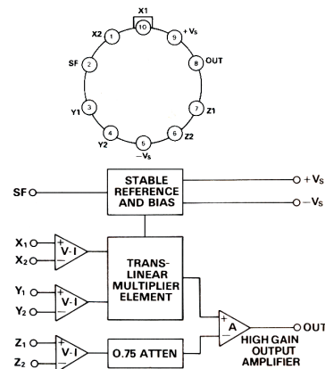
AD534JH
