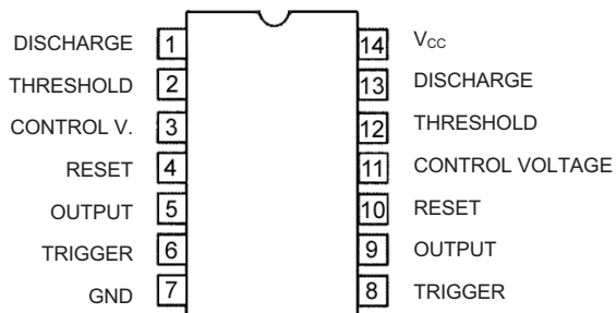
NE556
