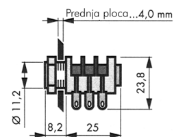
Typ S2 BBB Printmontage
