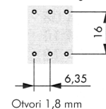
Typ S2 BBB Printmontage
