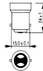
P13,5S
