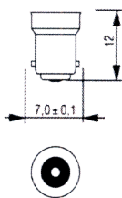
B22-2
