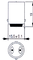
BA15
